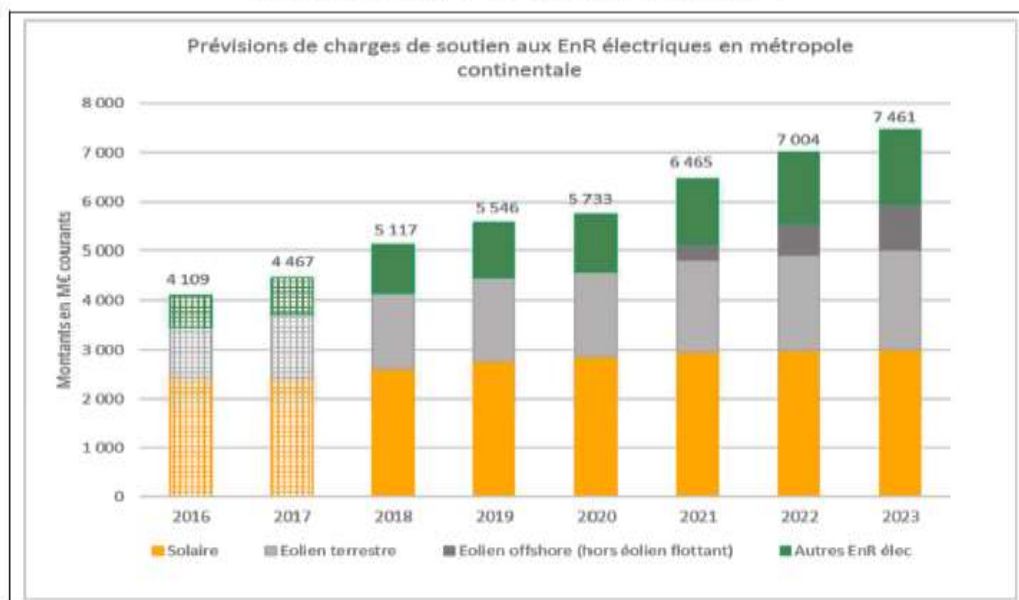
Graphique n° 11 : évolutions des charges de service public de l'énergie pour le soutien aux EnR électriques en métropole continentale
